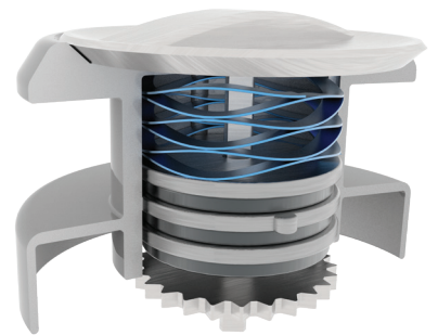
带有多层波形弹簧的旋转卷轴
