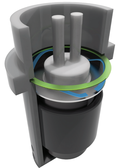
带平端波簧和螺旋挡圈的排气传感器
